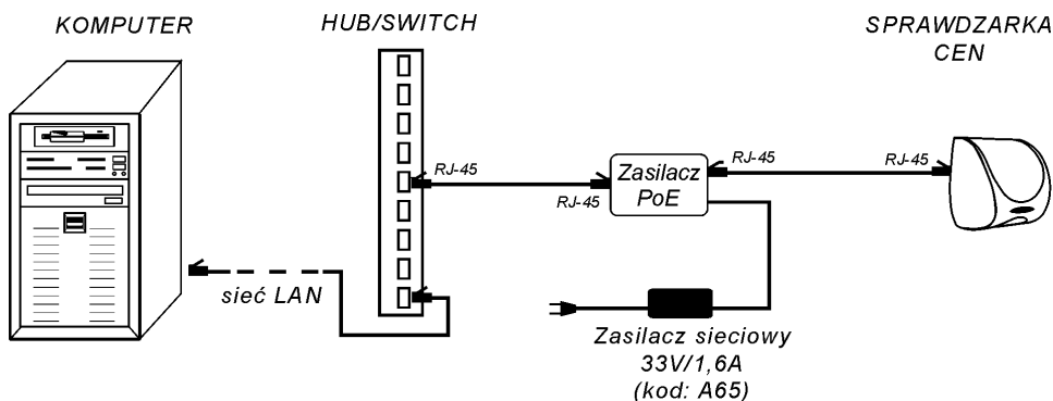
Rys. 5. Przykład połączenia pojedynczej sprawdzarki z zasilaczem PoE
